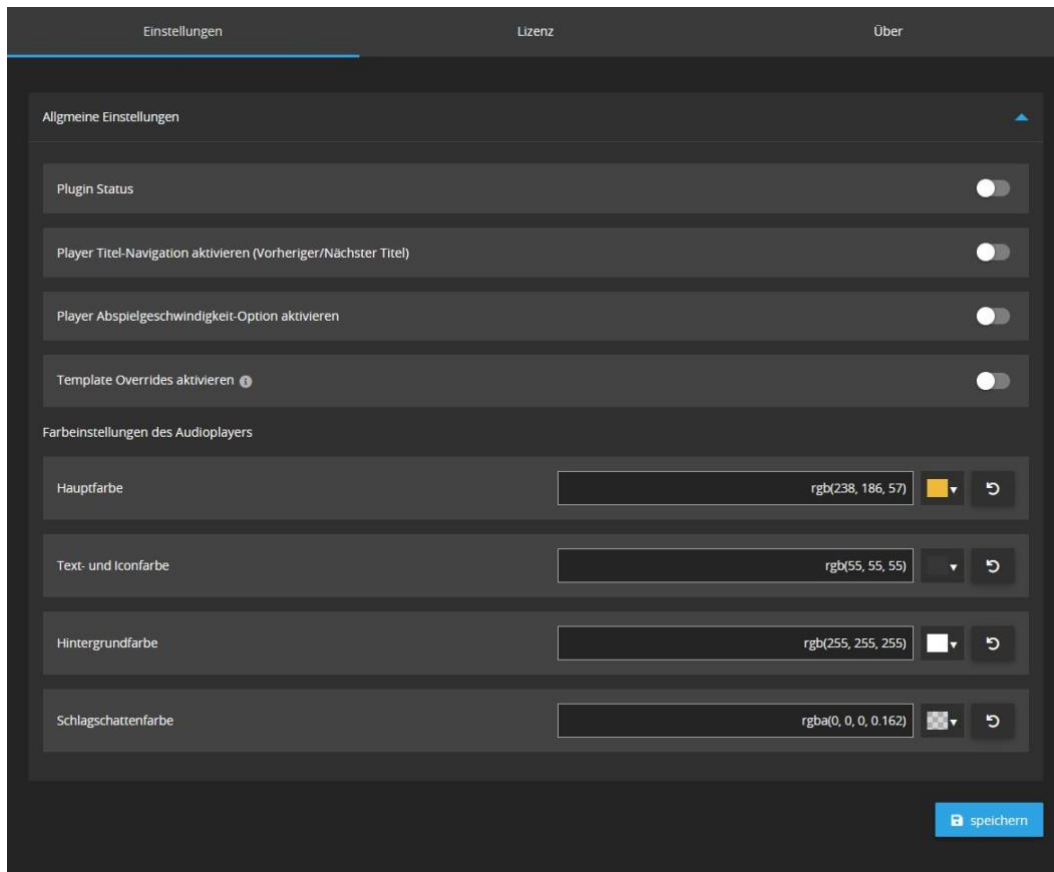
Abbildung 4: Reiter „Einstellungen“
