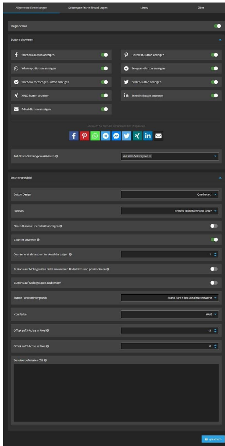
Abbildung 3: Reiter „Einstellungen“
